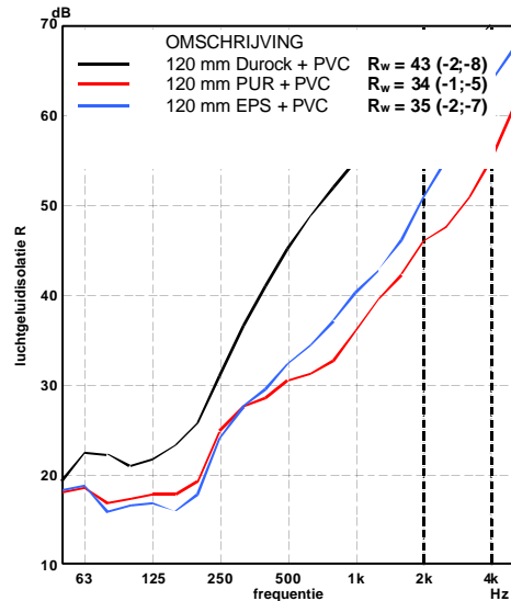
Prestaties steenwol versus kunststof isolatie
